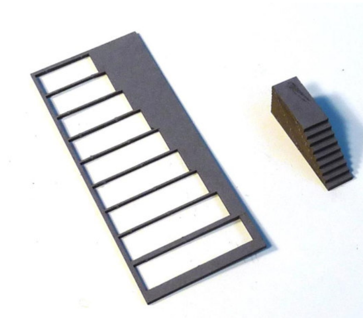
11. Treppe zusammenkleben
