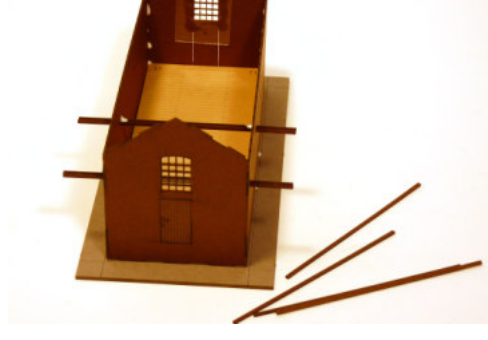
8. Dachsparren einkleben
