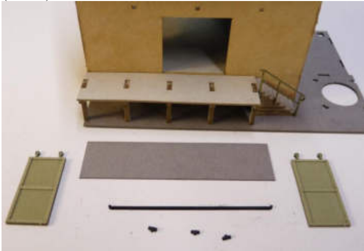
23. Tore aufkleben, eventuell Rest als Abstandshalter nutzen
