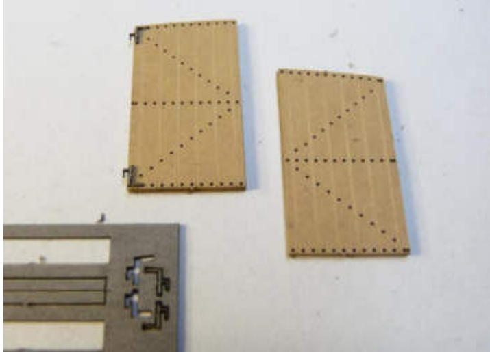
19. Beschläge außen in die Ecken kleben
