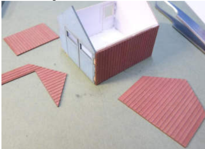
5. Türrahmen aufkleben, rechts bis Hausecke
